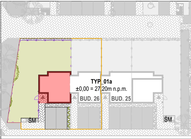
ZAGOSPODAROWANIE TERENU
