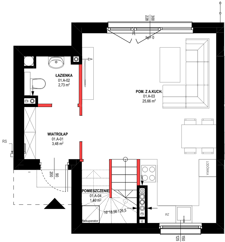
RZUT PARTERU
