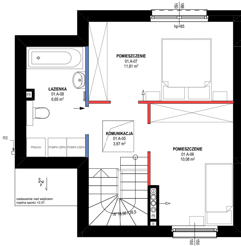
RZUT 1 PIĘTRA
